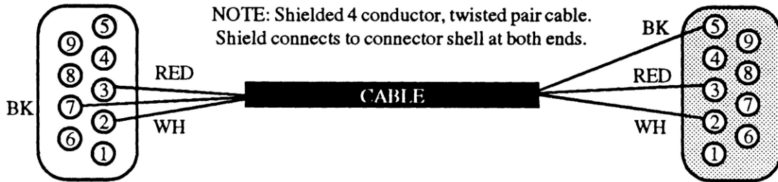
OMNI:CHRON II® - 9 PIN (MALE) PLUG
